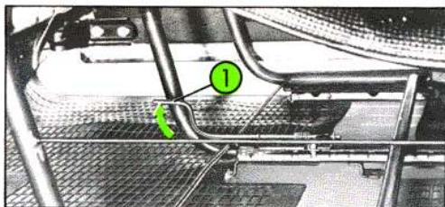
Fig. 11 Réglage banquette avant 1 - Manette de déverrouillage
