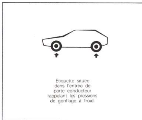
Fig. 3 Pression des pneumatiques
