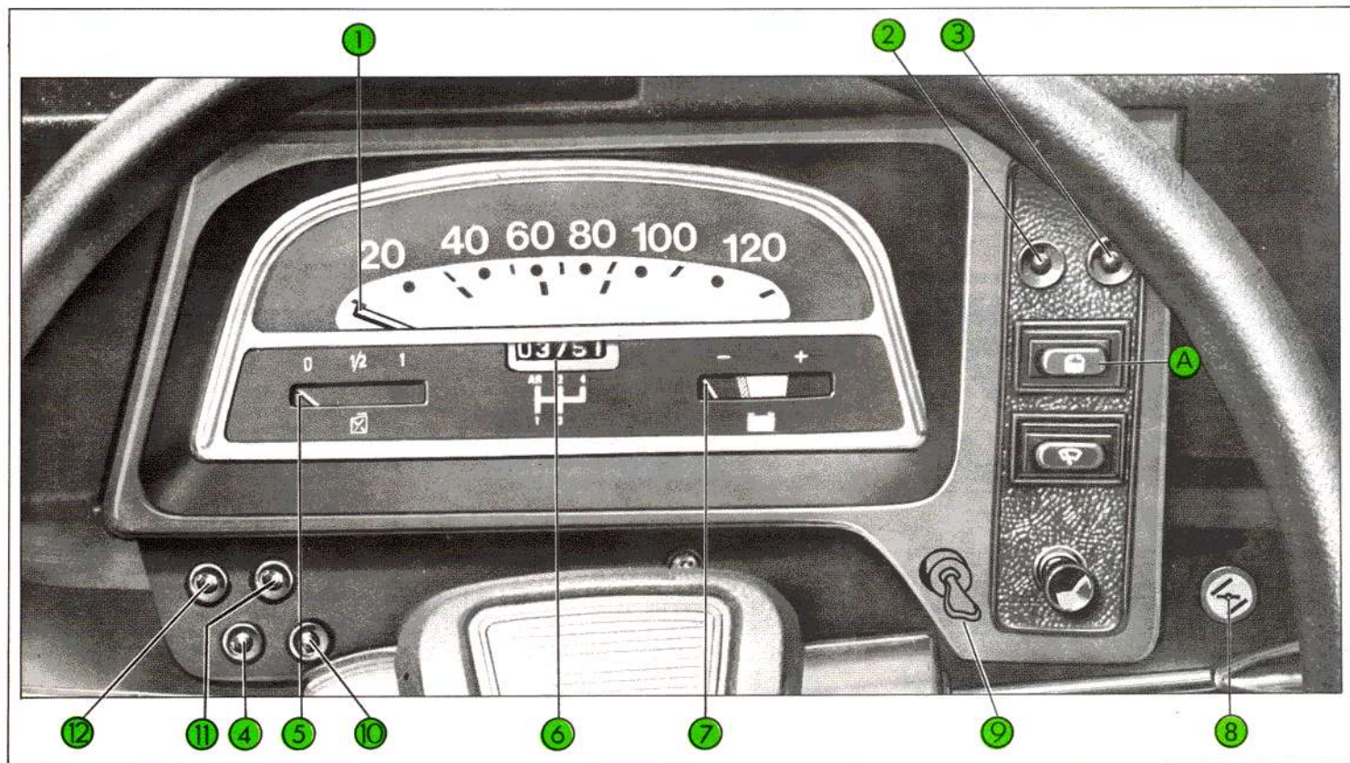
Fig 10 | Poste de conduite. Instruments de bord
