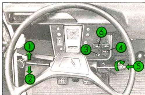
Fig. 22 Commande de signalisation
