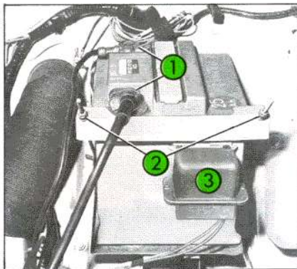
Fig. 11 Batterie 1 Bornes 2 Tirants 3 Régulateur
