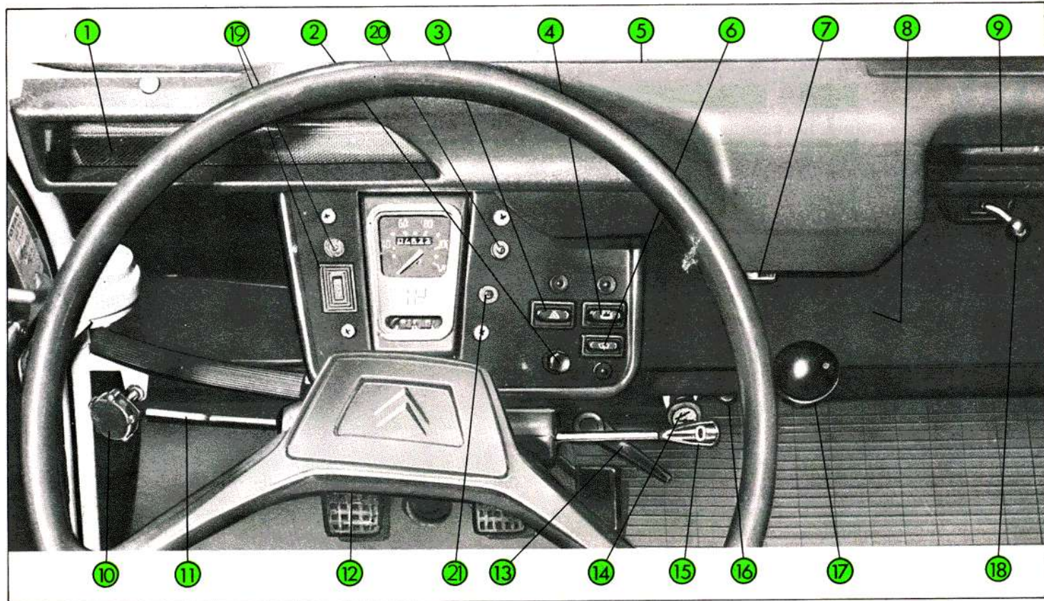
Fig 7 Poste de conduite : Commandes et accessoires
