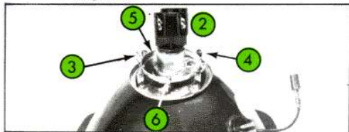
Fig. 7 Projecteurs « CIBIE »
