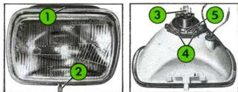
Fig. 5 Projecteurs « SEIMA »
