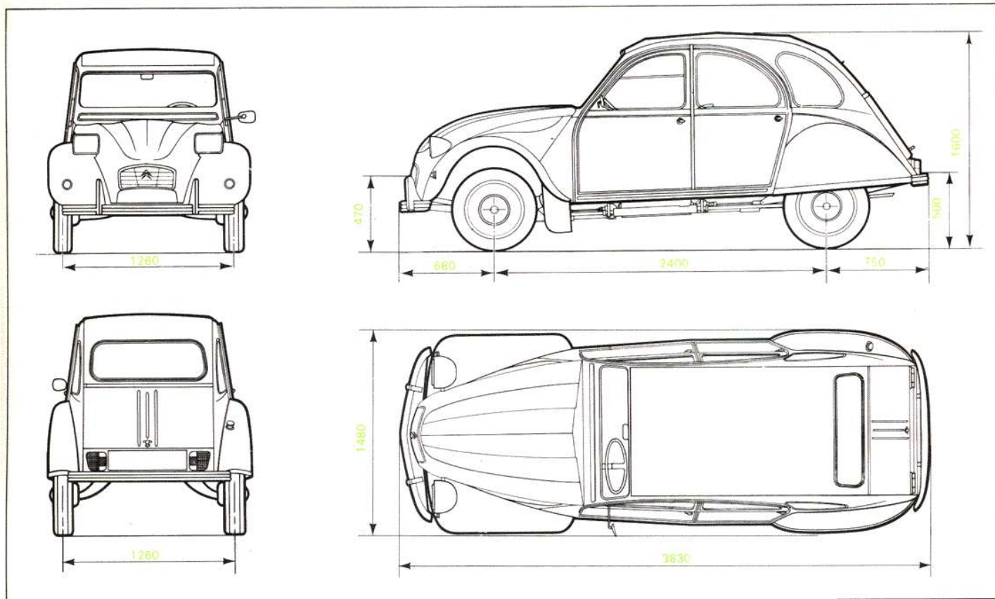
Fig. 3 Cotes d'encombrement
