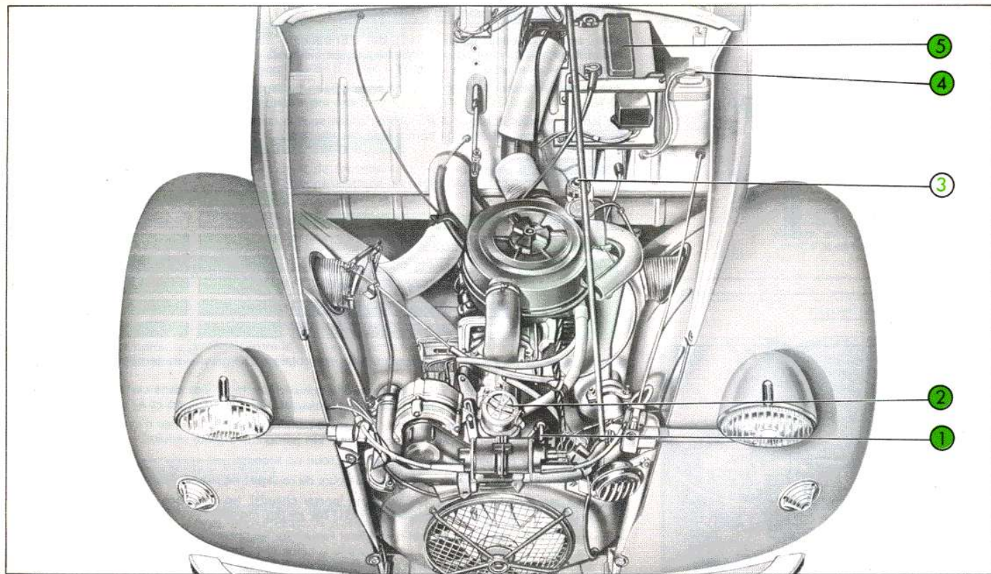
Fig. 2 Niveaux 1 - Jauge d'huile moteur 2 - Tubulure remplissage d'huile moteur 3 - Réservoir de liquide de frein 4 - Réservoir de lave-glace 5 - Batterie
