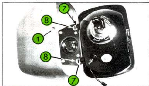
Fig. 6 Projecteurs « CIBIE »
