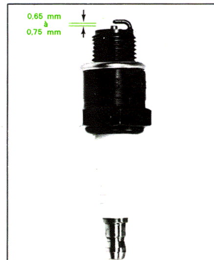
Fig. 12 Bougie : Ecartement des électrodes
