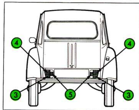
Fig. 5 | Eclairage extérieur et signalisation 3 - Indicateurs de direction arrière 4 - Stops 5 - Eclaireurs de plaque de police et feux de position arrière
