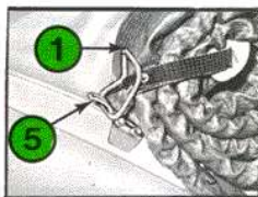
Fig. 30 Capote ouvrante 1 - Boucle extérieure 5 - Ergot de fixation arrière
