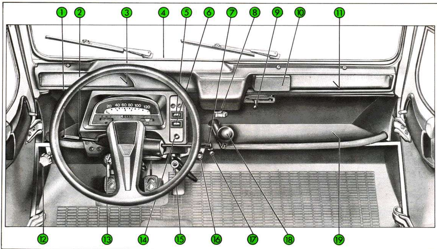
Fig. 8 Poste de conduite. Commandes et accessoires
