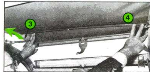
Fig. 32 Ouverture avant de la capote 3 - Cadre 4 - Traverse
