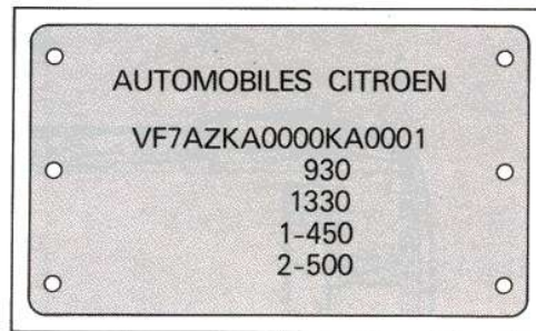
Fig. 1 Plaque constructeur
