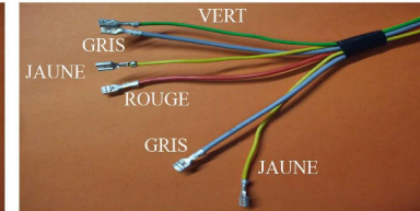
INTERRUPEUR WARNING
